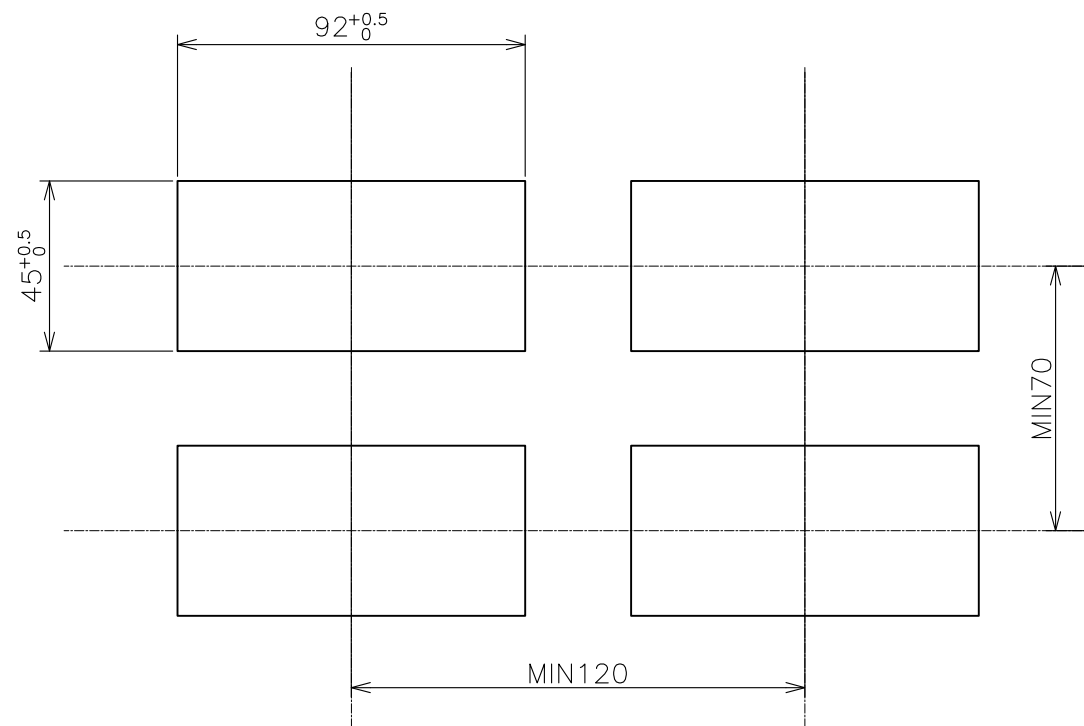
パネルカット Panel cut
