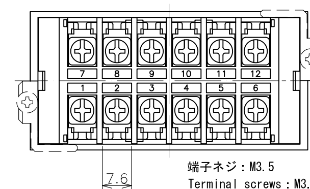
後部端子 rear side (terminal part)
