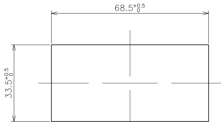
パネルカット Panel cut-out dimension
