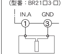
□マグネチックセンサ (型番: BR21□3-□)
