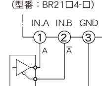
□ラインドライバ (型番: BR21□4-□)
