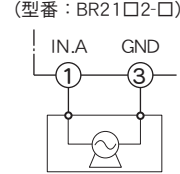
□ACタコジェネ (型番: BR21□2-□)
