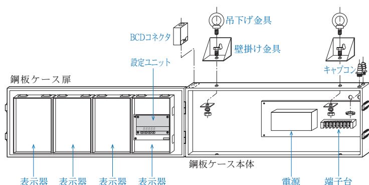
＜例＞HS231S-4A21（ケース扉開時の内部構成図）
