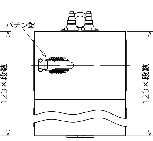
□HS122W（両面）
