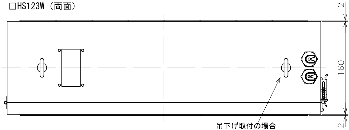
□HS123S（片面）
