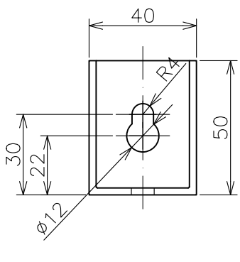
（参考寸法）
