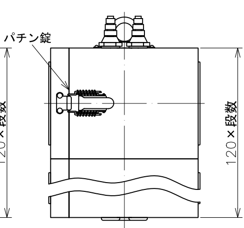
□HS123W（両面）
