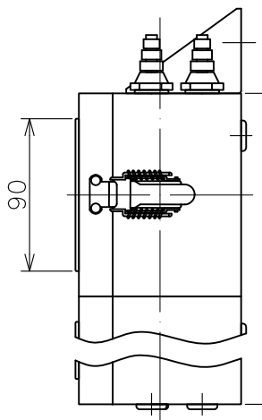
□HS122S（片面）
