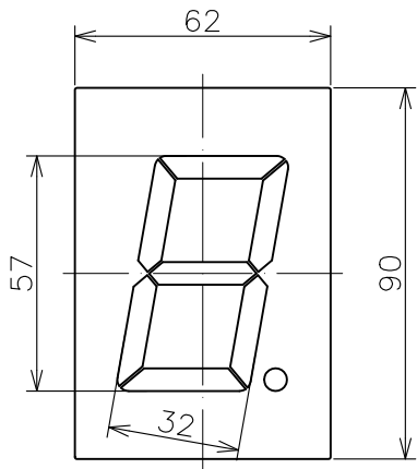
尺度1/2
