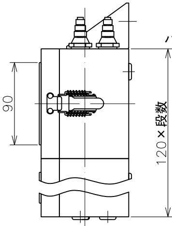
□HS121S（片面）
