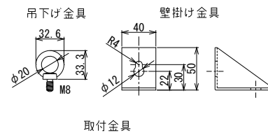
取付金具
