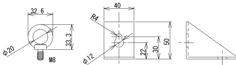
取付金具
