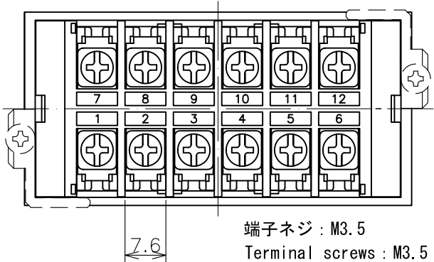
後部端子 rear side (terminal part)
