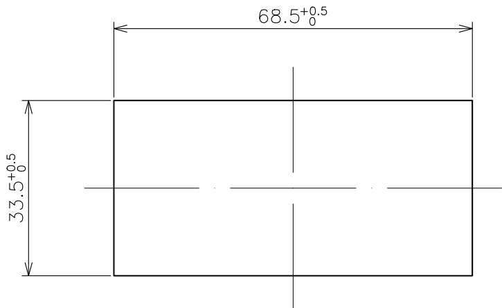
パネルカット Panel cut-out dimension
