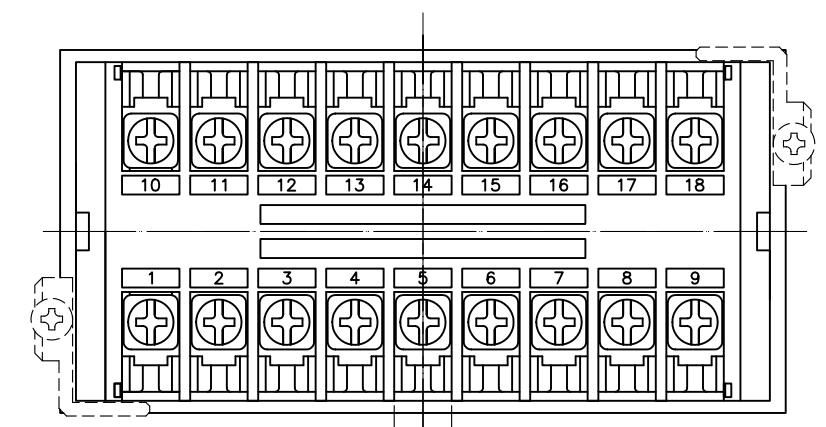
端子ネジ : M3.5 Terminal screws : M3.5
