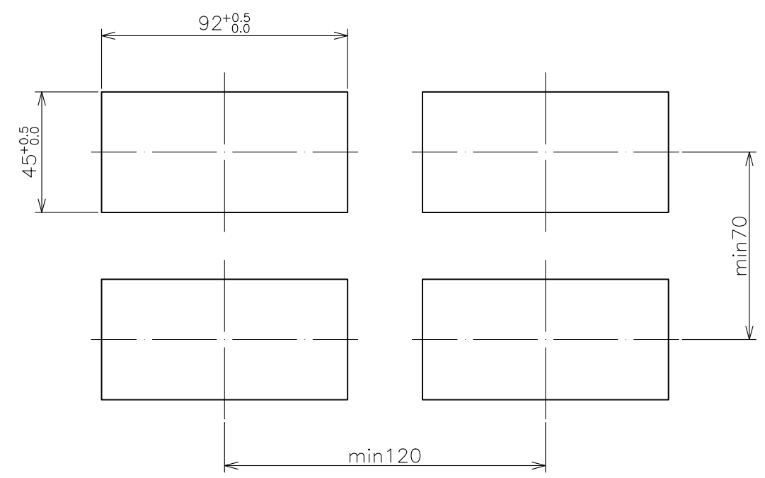
パネルカット Panel cut-out dimension
