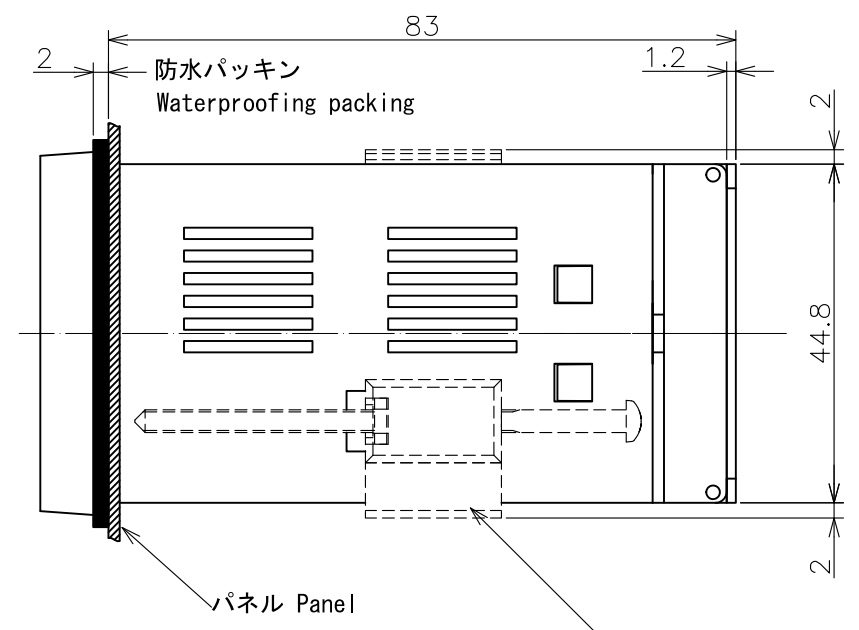
取付具 (固定ネジ : M3) Fixture (Fixed screw : M3)
